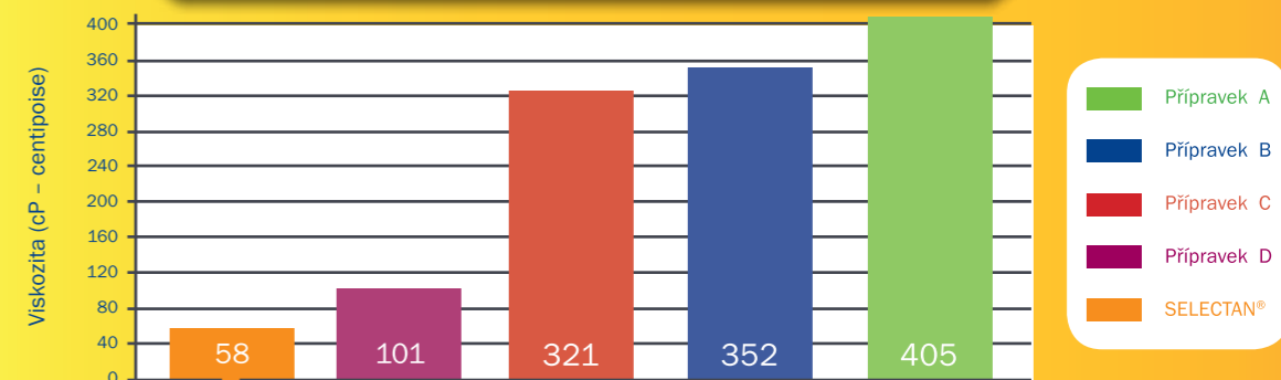
Porovnání viskozity (nízká teplota) 5 °C + 3 °C
